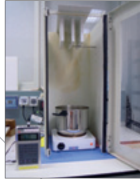
Figura 47. Resistenza al vapore: metodo AMK.
