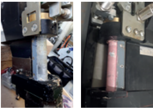
Figura 68. Esempi di testine con adesivo poliuretano reticolato.
