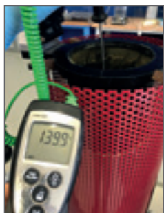
Figura 50. Sonda ad immersione.
