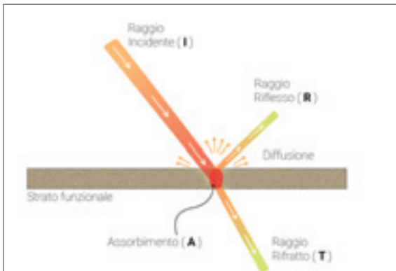
Figura 36. Schematizzazione dell'interazione tra raggio laser e bordo.
