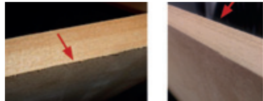
Figura 73. Esempio di pannello con linea di taglio rovinata da utensile usurato.
