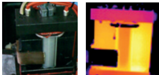
Figura 61. Immagine del rullo: a sinistra in scala di grigi; a destra termografica.
