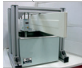
Figura 48. Resistenza al vapore: metodo secondo capitolato di un produttore di mobili.
