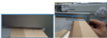
Figura 75. Esempio di pannello alto 45 mm rettificato con frese non in squadro.
