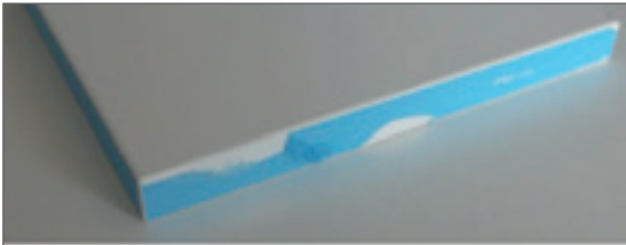
Figura 82. Esempio di bordo con pellicola rimossa dai copiatori frontali dell'arrotondatore.
