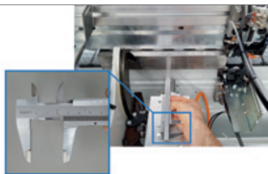
Figura 78. Esempio di misura della linea di lavoro: distanza tra la superficie laterale del pannello ed il supporto del cingolo misurata con il calibro.
